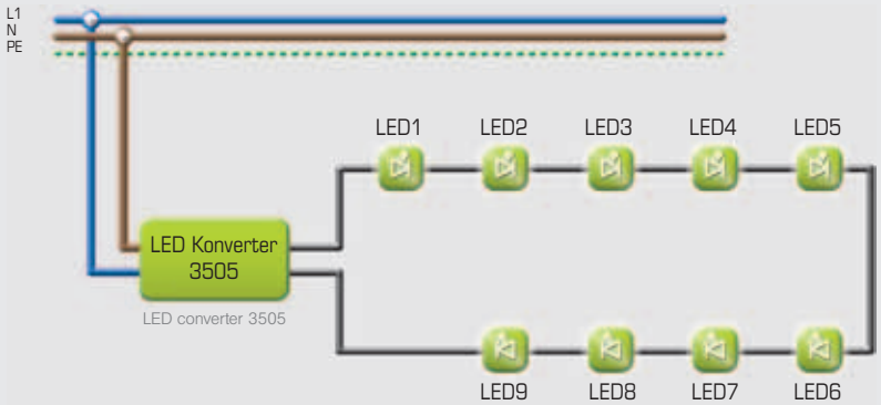
Reihenschaltung, max. Leitungslänge sekundärseitig 20m series connexion, max. length of connection cable secondary side 20m
