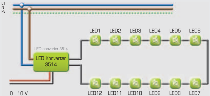
Reihenschaltung, max. Leitungslänge sekundärseitig 10m series connexion, max. length of connection cable secondary side 10m
